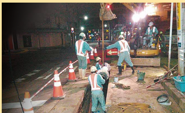
▲城内町の耐震管布設工事
