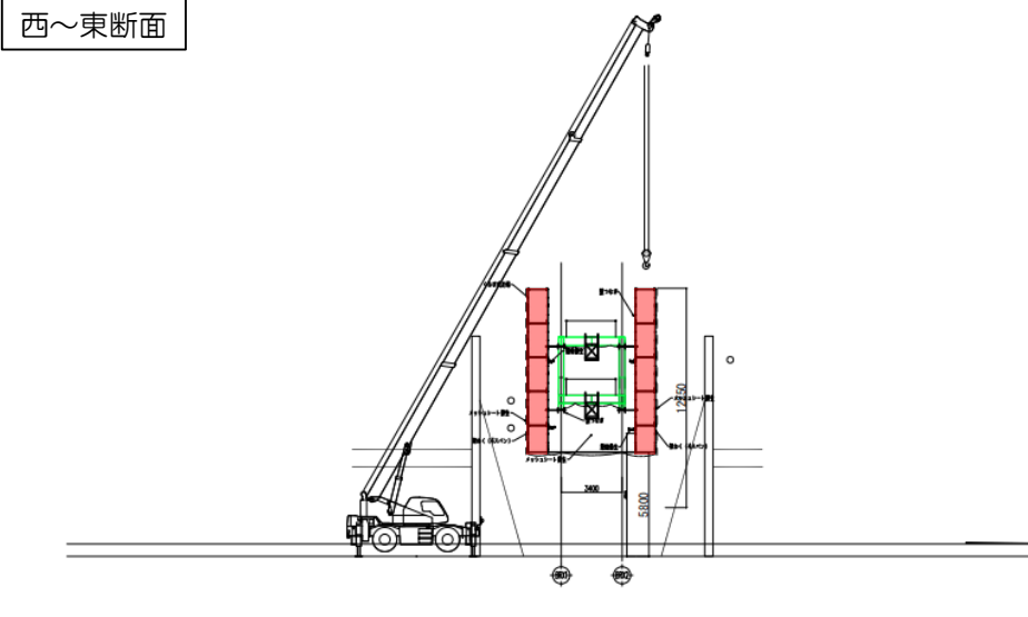
南～北断面
