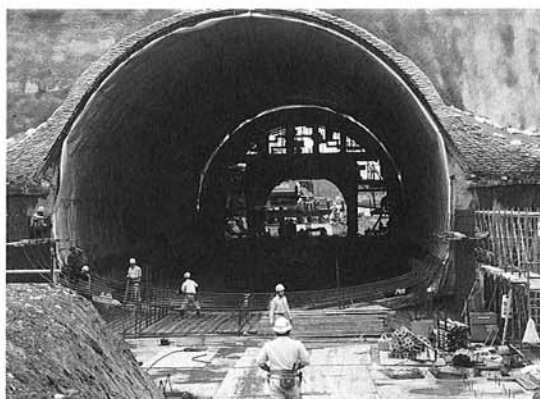
▲116号バイパス・八幡林トンネル工事風景
