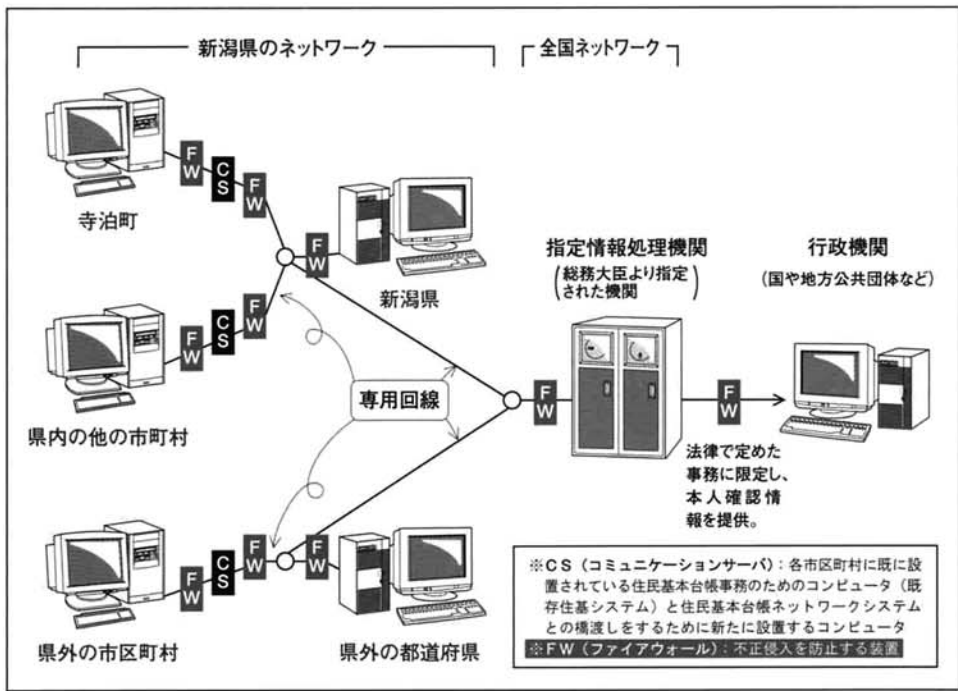
役場に設置された住民基本台帳事務のためのコンピュータ (CS・FWなど)
