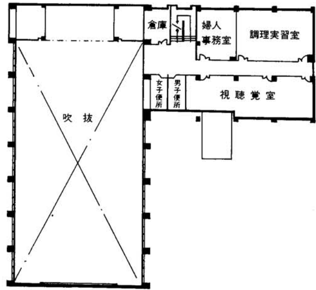
2F平面図
