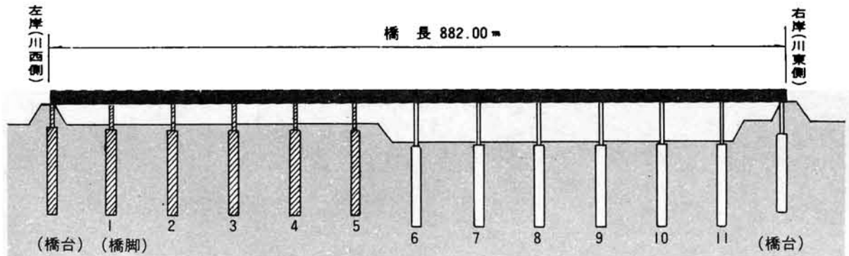
この部分の橋台と橋脚の工事を昭和55年度に行います。
