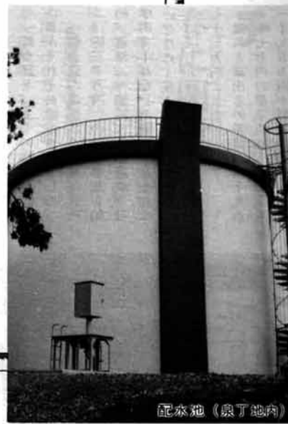
町にある半地下式の配水池 直径は一・三メートル。容量は四百トン。隣りに容量三百トンのもう一基の配水池もある。
