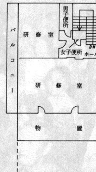
2階平面図
