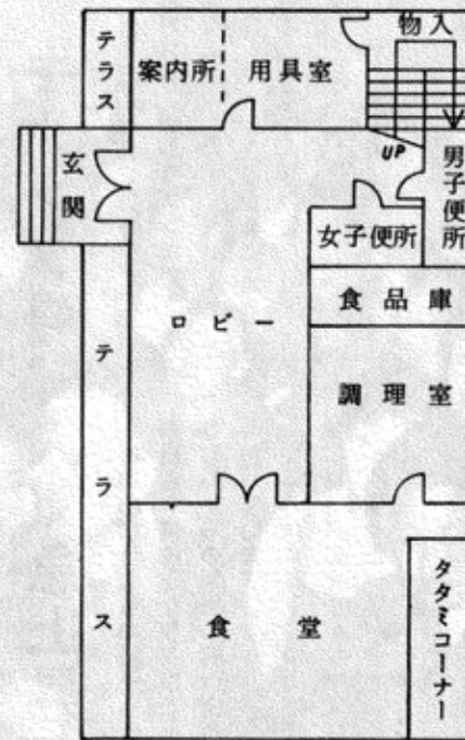
1階平面図
